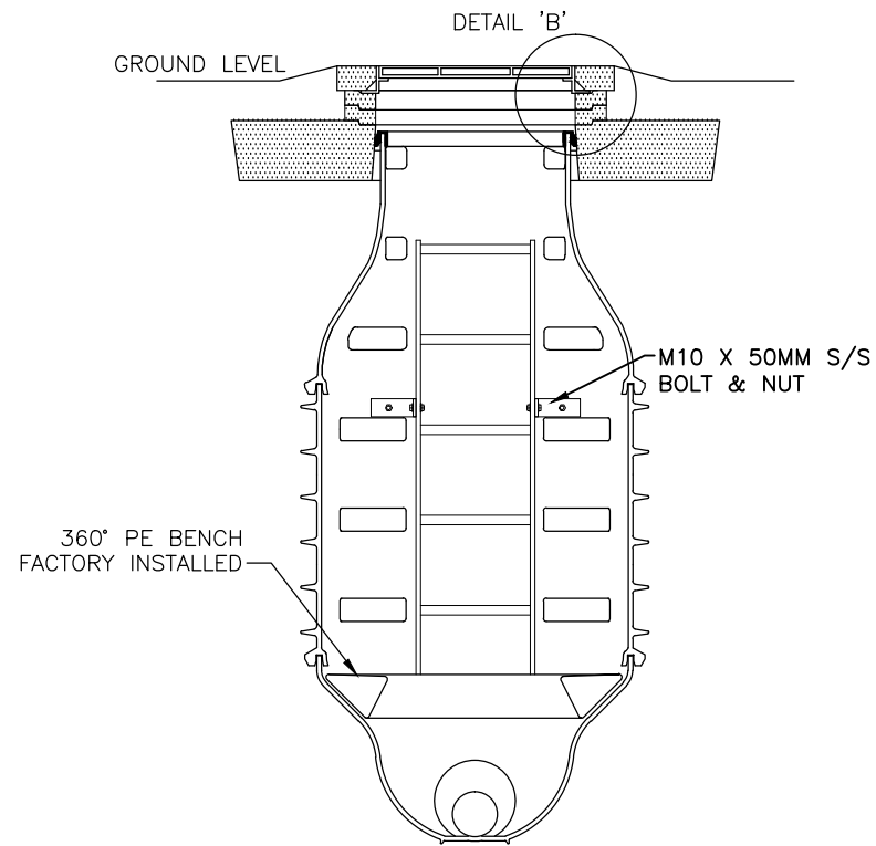
SECTION 'B-B'
